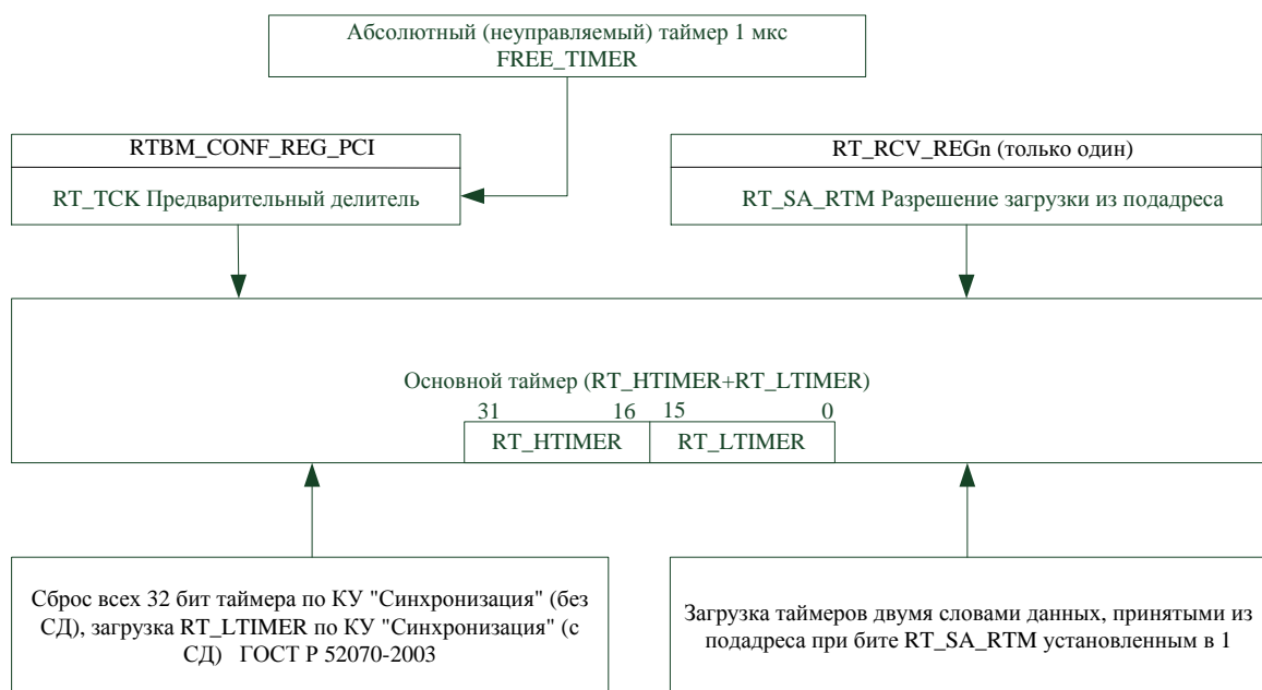
Рисунок 8. Организация таймеров для каждого канала в режимах ОУ и АМШ.
