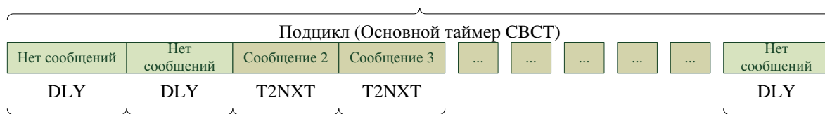
Рисунок 7. Связь таймеров внутри подцикла с заменой неиспользуемых сообщений таймером DLY .
