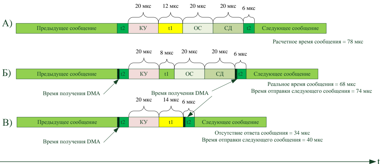
Рисунок 15. Сообщения без использования таймера T2NXT.
