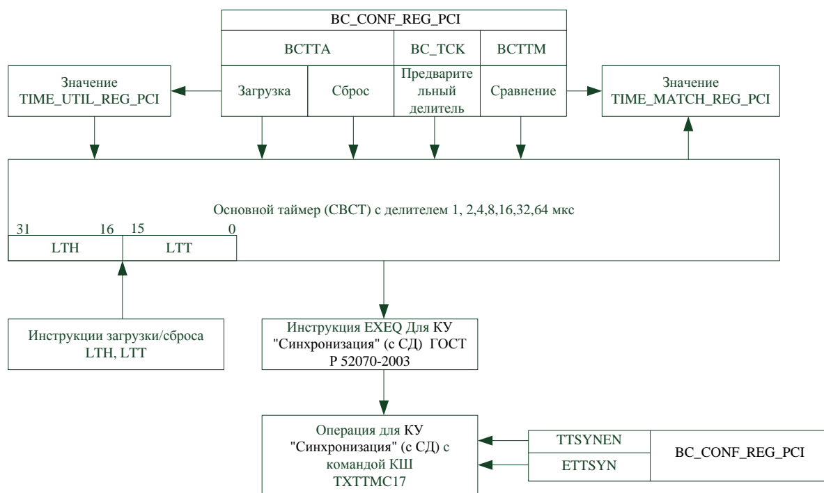
Рисунок 8. Структура основного таймера КШ (CBCT).
