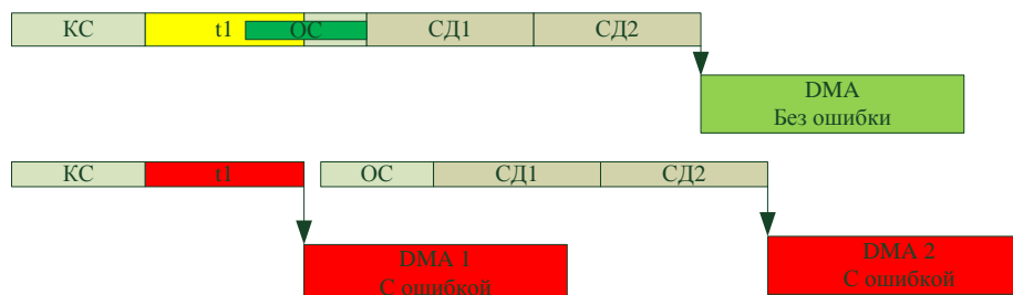
Иллюстрация превышения интервала t1 для примера 2.
