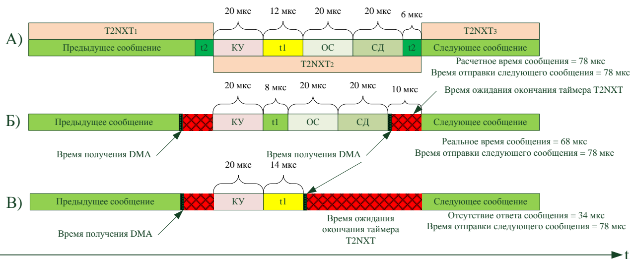
Рисунок 12. Использование таймера T2NXT с параметрами по умолчанию.
