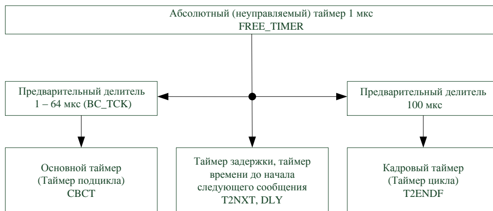
Рисунок 4. Организация таймеров для каждого канала в режиме КШ.
