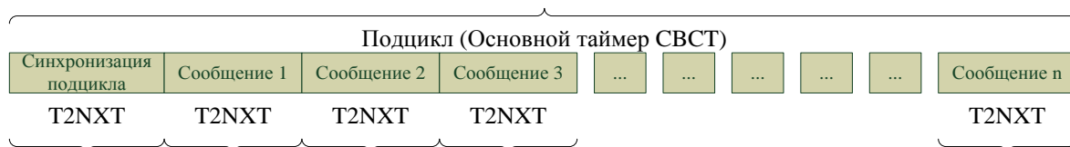
Рисунок 6. Связь таймеров внутри подцикла, состоящего из последовательности сообщений до конца подцикла без интервалов свободного времени.
