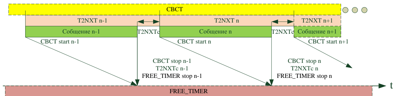
Рисунок 13. Связь таймеров в сообщениях DMA.
