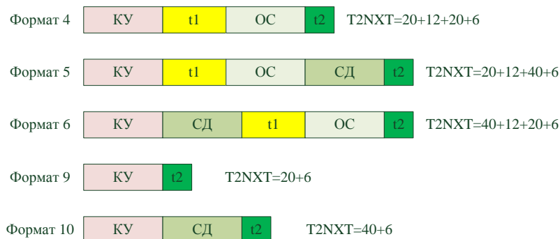
Рисунок 11. Форматы с постоянной длиной данных.
