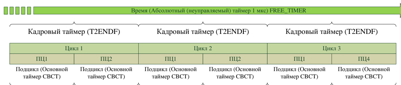
Рисунок 5. Связь таймеров для нескольких циклов.
