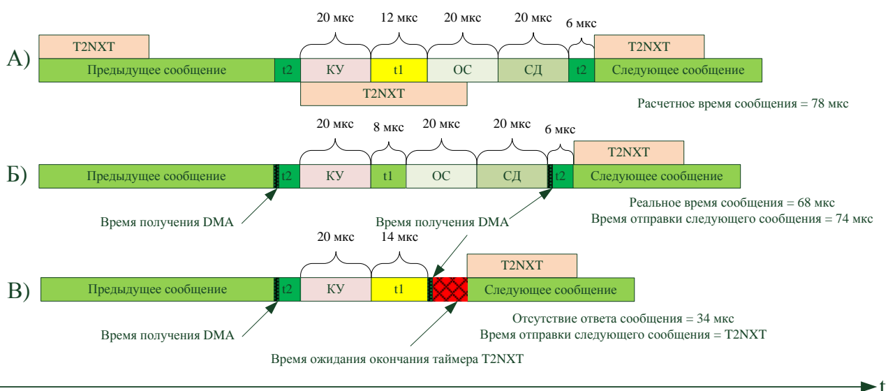
Рисунок 14. Использование таймера T2NXT со значением меньше длины сообщения.
