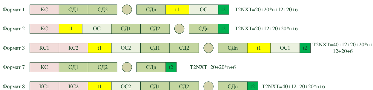
Рисунок 10. Форматы с переменной длиной данных.
