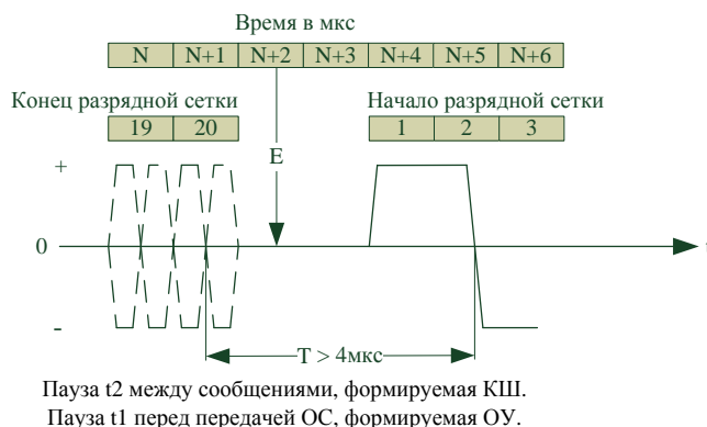
Рисунок 9. Пауза между сообщениями и пауза перед передачей ОС.
